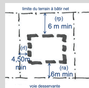
Fig. 25 : Recul antérieur (ra), latéral (rl) et postérieur (rp)
