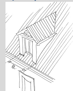
Fig. 52 : Autres lucarnes : \ell \leq 1,50\text{m}
