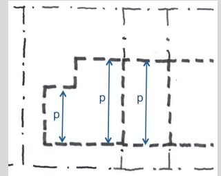
Fig. 12b : Profondeur en cas de maisons accolées (p)
