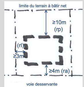
Fig. 15 : Recul antérieur (ra), latéral (rl) et postérieur (rp)
