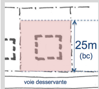
Fig. 13 : Bande de construction (bc)
