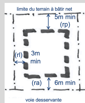
Fig. 38 : Recul antérieur (ra), latéral (rl) et postérieur (rp)
